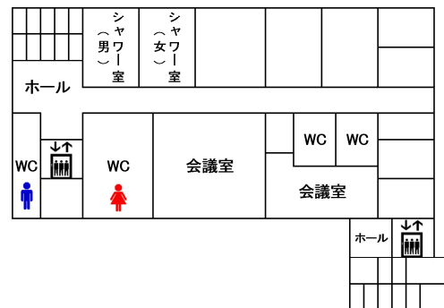
地下1階
