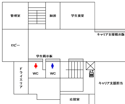
1階
